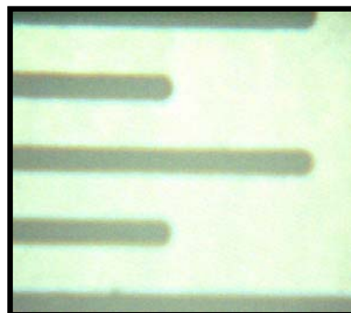
最大検出範囲 2.0mm x 2.9mm 1目盛0.5mmのスケールを撮像している。 設置距離 11mm Maximum sensing range is 2.0mm x 2.9mm . Showing a 0.5mm scale. Setting distance is 11mm.
