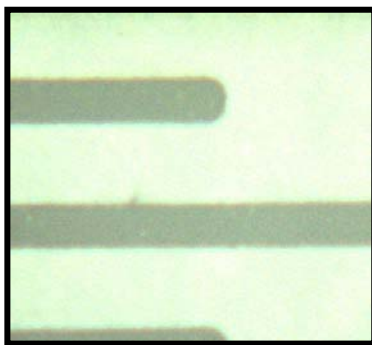
最小検出範囲 1.5mm x 2.0mm 1目盛0.5mmのスケールを撮像している。 設置距離 9mm Minimum sensing range is 1.5mm x 2.0mm . Showing a 0.5mm scale. Setting distance is 9mm.
